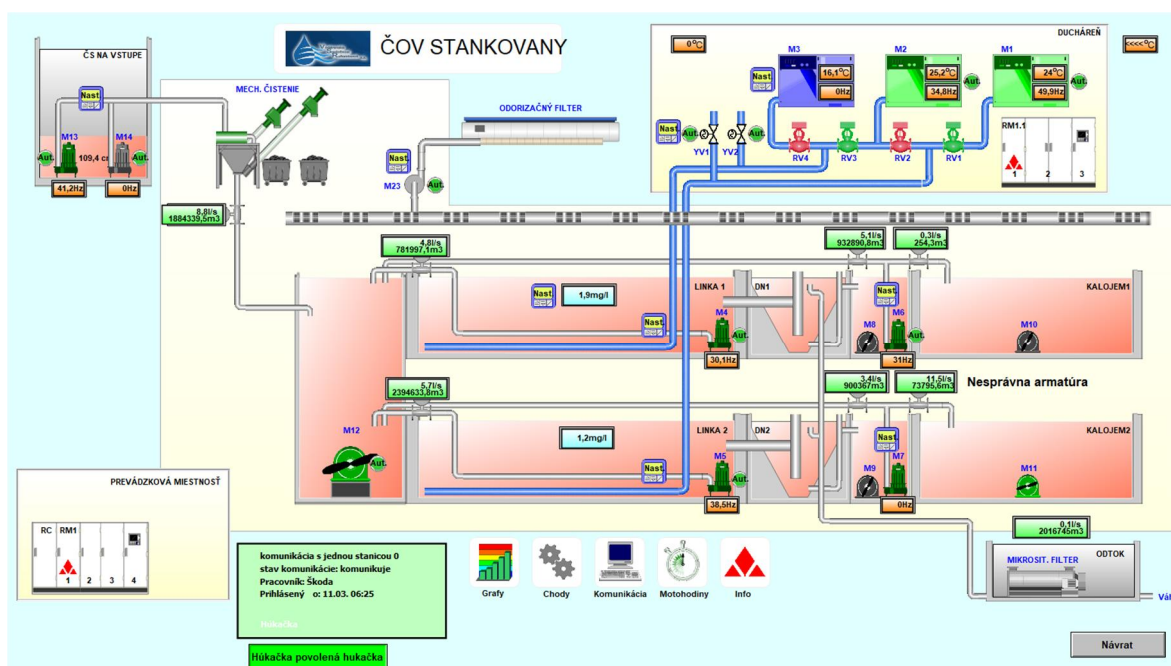
Obr. Dispečingový systém – Snímanie chodu ČOV Rojkov
