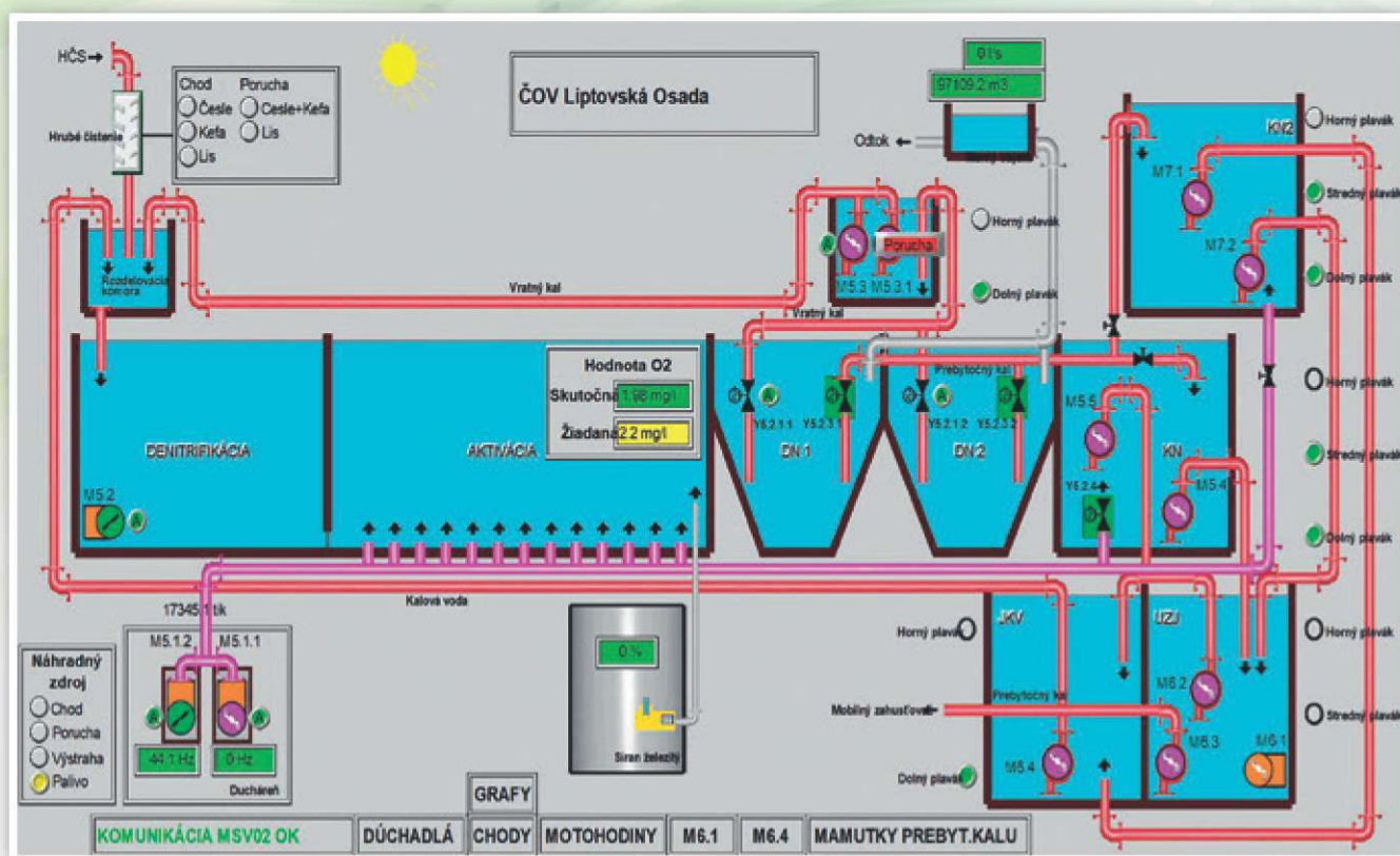
Dispečingový systém – Blokova schéma ČOV Liptovská Osada
