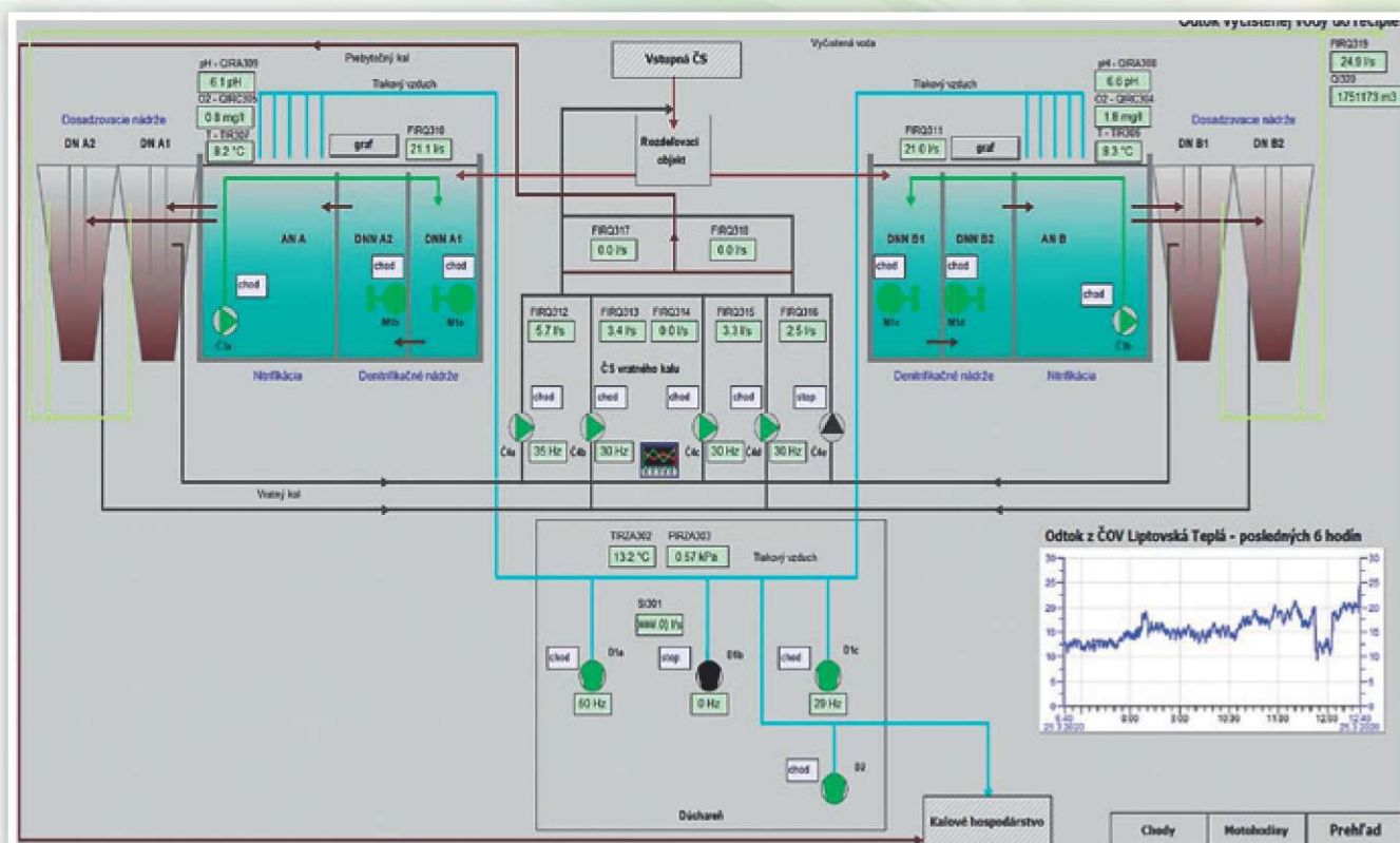
Dispečingový systém – Bloková schéma ČOV Liptovská Teplá
