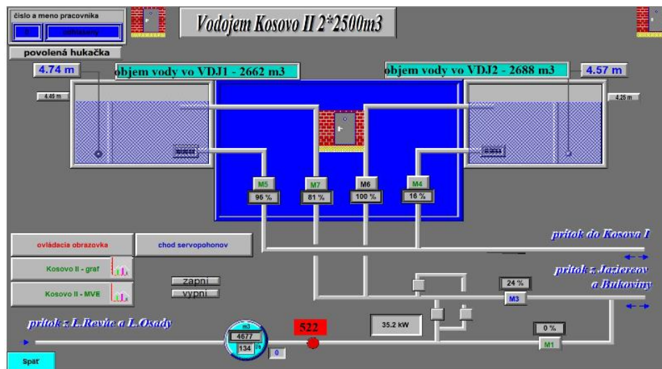
Obr. Dispečingový systém – Bloková schéma VDJ Kosovo II
