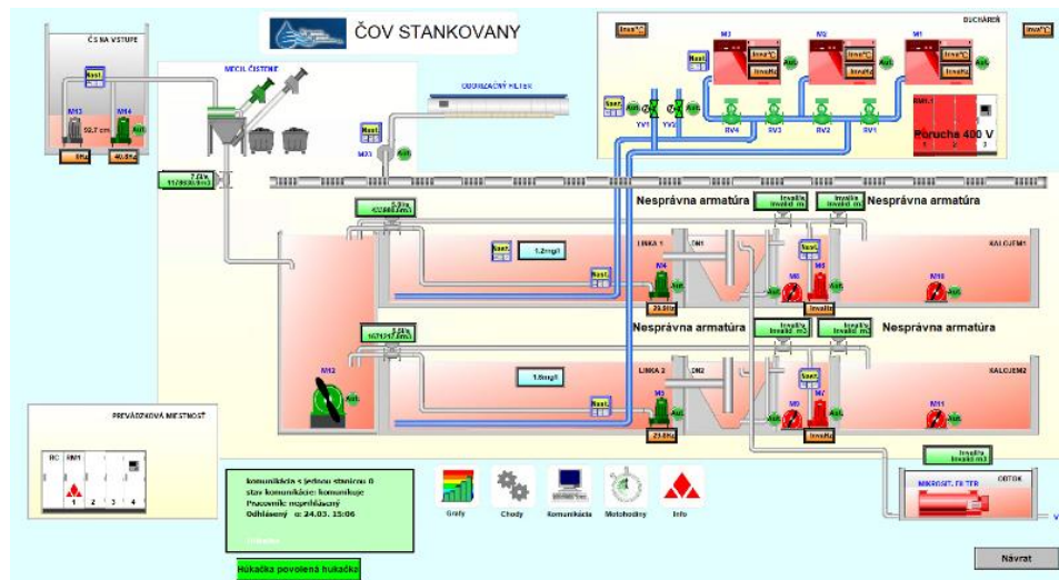
Obr. Dispečingový systém – Blokovaná schéma ČOV Rojkov
