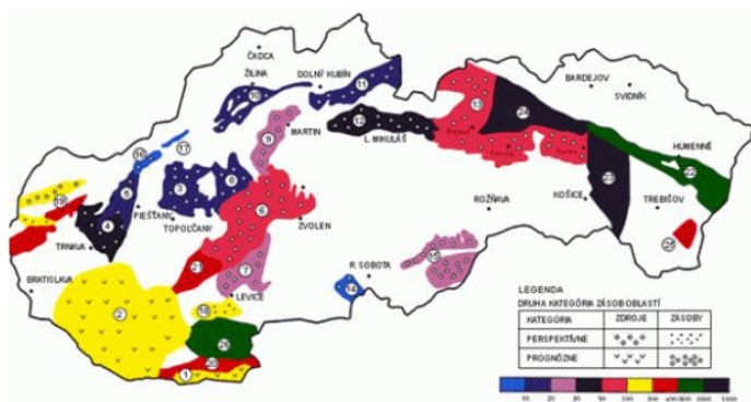
Geotermálna energia a jej využívanie na Slovensku
