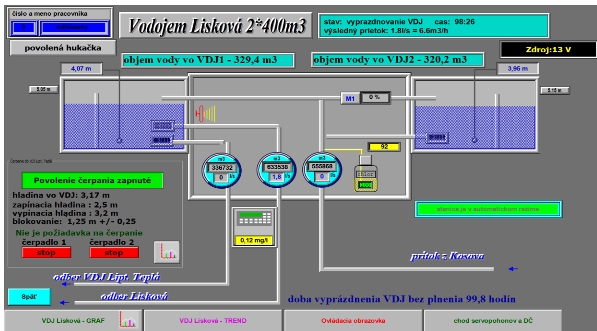
Obr. Dispečingový systém – Blokova schéma VDJ Lisková (2x400m 3 )
