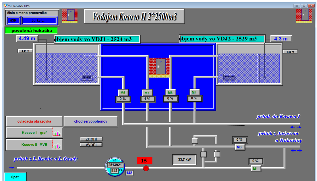
Obr. Dispečingový systém – Sledovanie prevádzky vodojemu Kosovo v Ružomberku
